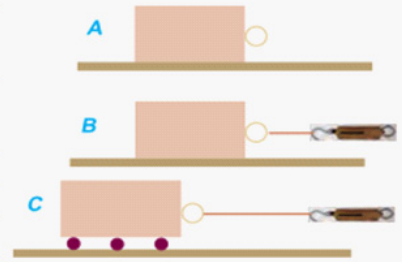
चित्र 6. 10 घर्षण घटाउने उपाय
